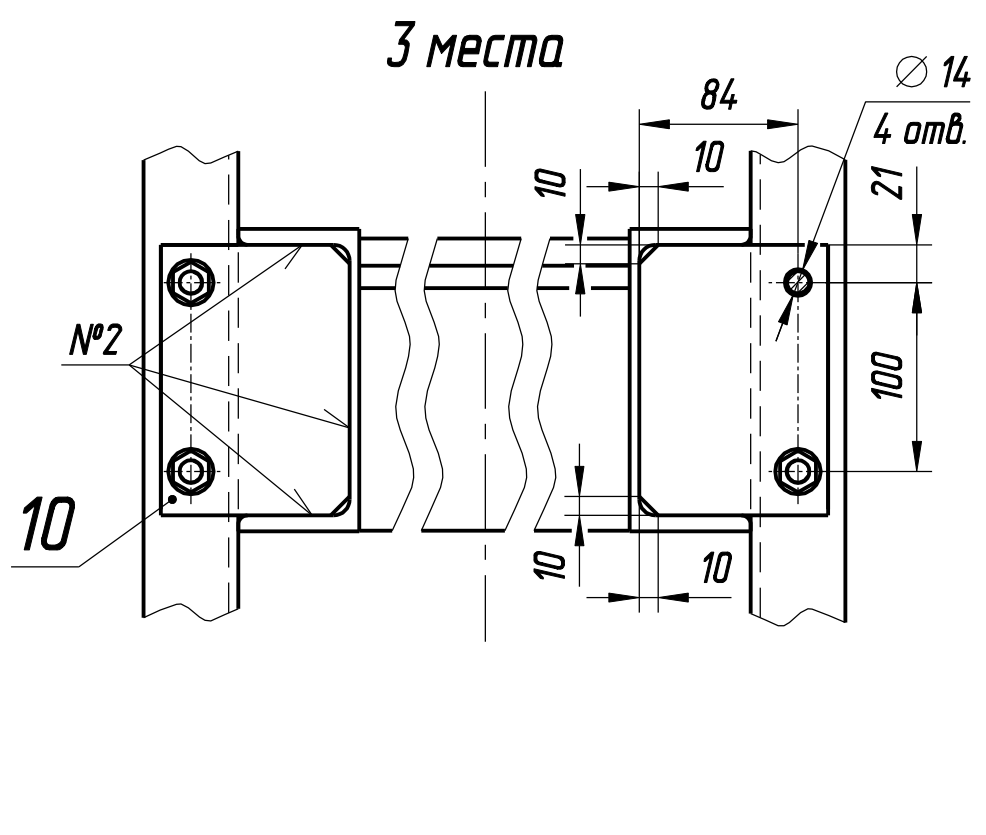
Е (1:2)
