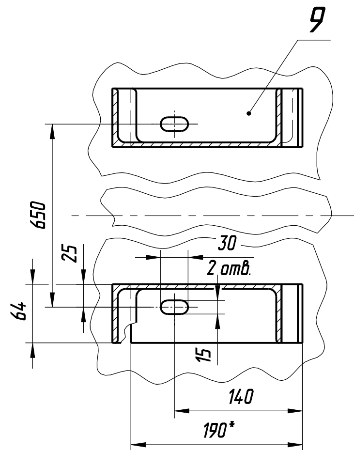
Б-Б (1:4)
