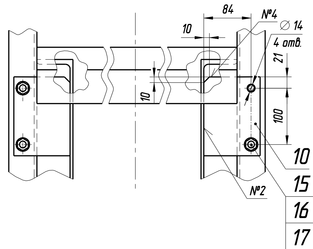
Д (1:2)
